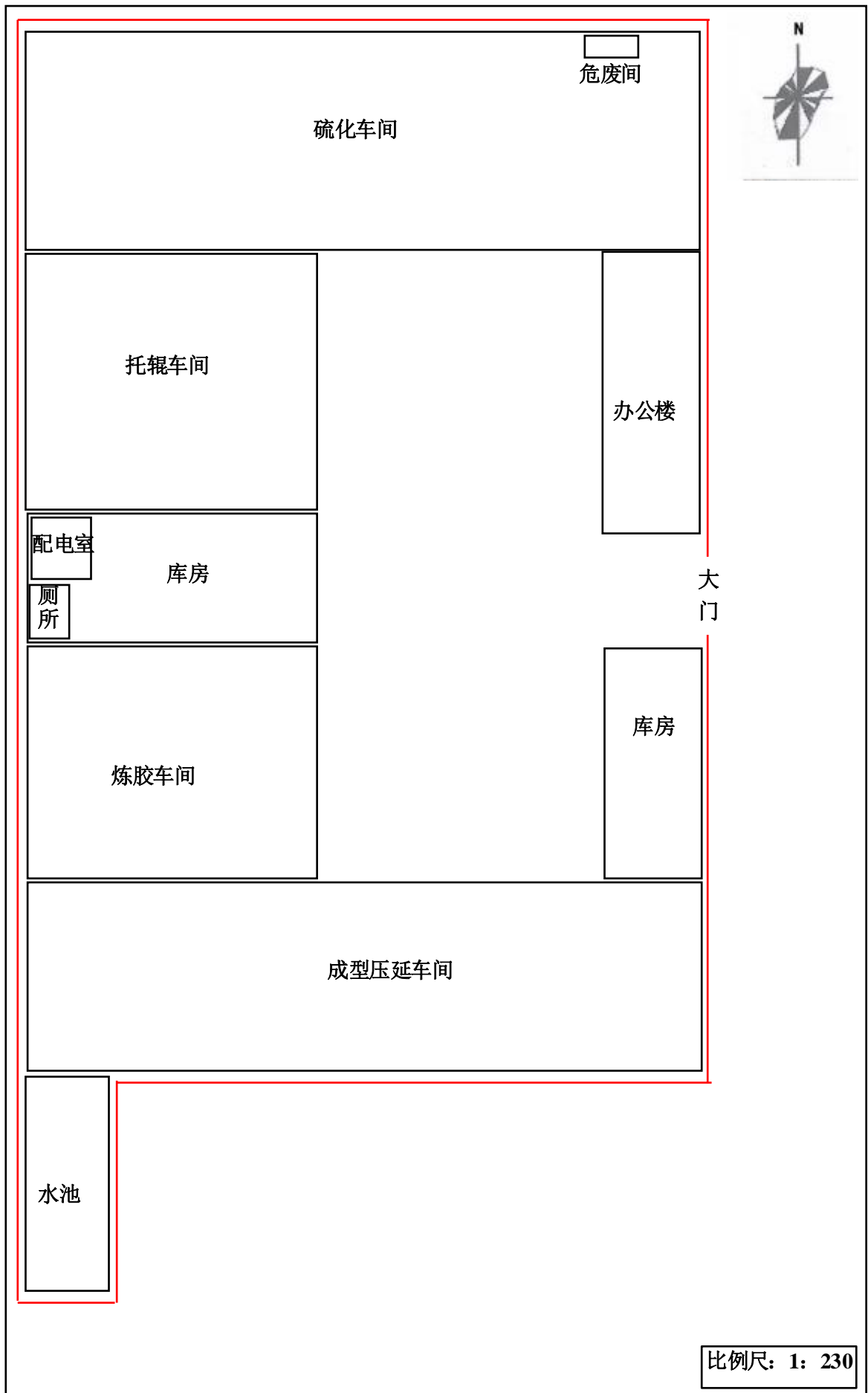
附图 4 建设项目厂区平面布置示意图
